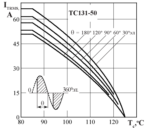
Рисунок 2 - Зависимость допустимого действующего тока в открытом состоянии I_{TRMS} от температуры корпуса T_c для токов синусоидальной формы частоты f = 50 Гц
