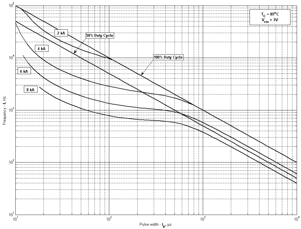
Рис. 11 – Зависимость частоты синусоидальных импульсов тока от длительности импульсов
