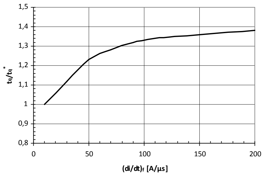
Рис. 4 — Зависимость времени выключения t_q от скорости спада анодного тока di/dt
