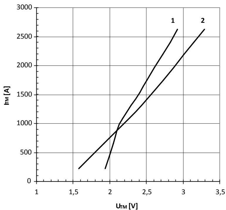
Рис.1 – Предельная вольт-амперная характеристика.
