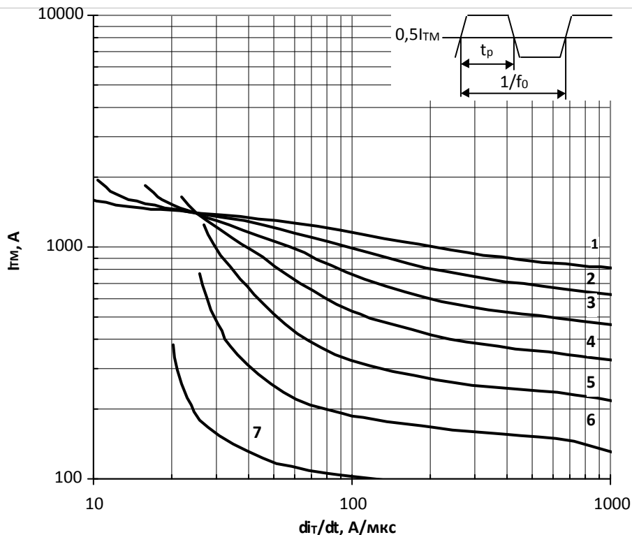
Рис. 13 – Зависимость импульсного тока в открытом состоянии I_{TM} трапецевидной формы тока от скорости нарастания тока di_T/dt для длительности импульсов t_p=1/4f_0 и температуры корпуса T_c=65^\circ\text{C} на высоких частотах.
