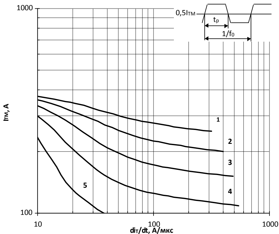
Рис. 12 – Зависимость импульсного тока в открытом состоянии I_{TM} трапециевидной формы тока от скорости нарастания тока di_T/dt для длительности импульсов t_p=1/2f_0 и температуры корпуса T_c=105 °С на высоких частотах.
