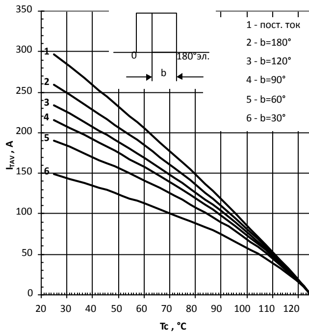
Рис. 5 – Зависимость максимально допустимого среднего в открытом состоянии тока I_{TAV} от температуры охлаждения T_c для охлаждающего воздушного потока 6 м/с, радиатор О143 и прямоугольной формы тока при различных углах проводимости, f=50 Гц.
