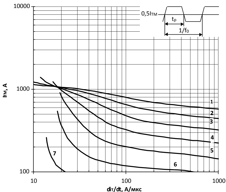
Рис. 14 – Зависимость импульсного тока в открытом состоянии I_{TM} трапецевидной формы тока от скорости нарастания тока di_T/dt для длительности импульсов t_p=1/4f_0 и температуры корпуса T_c=85^\circ\text{C} на высоких частотах.
