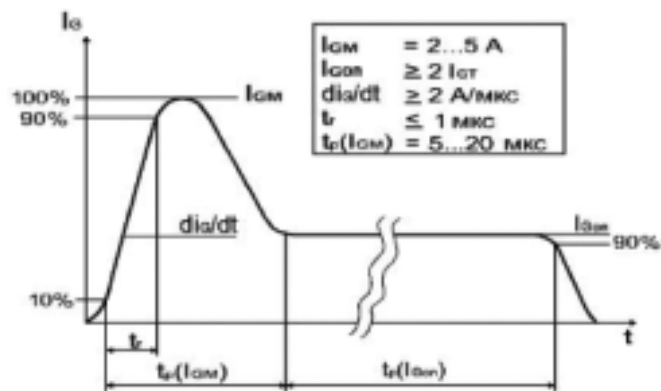
Рисунок 13: Рекомендуемая форма импульса управления. t(I_{с(м)}) - определяется характеристиками тиристора и режимом работы преобразователя.
