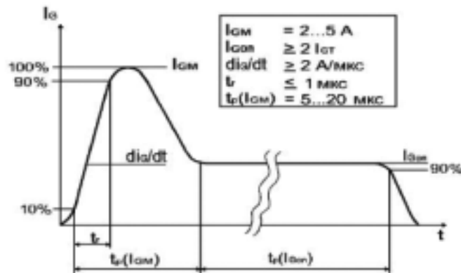
Рисунок 13: Рекомендуемая форма импульса управления. t(I_{с(п)}) - определяется характеристиками тиристора и режимом работы преобразователя.
