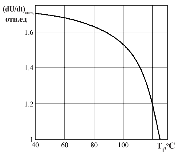
Рисунок 12 - Зависимость критической скорости нарастания коммутационного напряжения (dU_D/dt)_{com} (н.е.д.) от температуры структуры T_j при I_T = I_{TRMS} , t_i = 10\text{ мс} .
