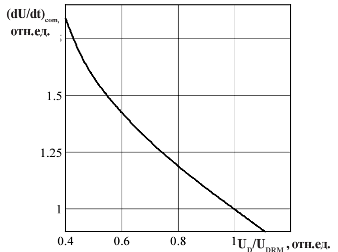
Рисунок 13 - Зависимость критической скорости нарастания коммутационного напряжения (dU_D/dt)_{com} (н.ед.) от величины приложенного напряжения U_D/U_{DRM} (н.ед.) при I_T = I_{TRMS} , T_j = 125^\circ\text{C} , t_i = 10\text{ мс} .
