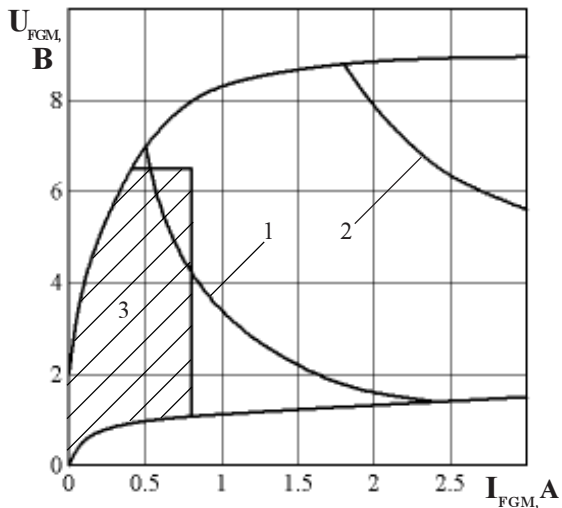
Рисунок 9 - Предельные характеристики цепи управления
