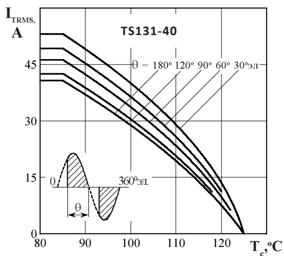
Рисунок 2 - Зависимость допустимого действующего тока в открытом состоянии I_{TRMS} от температуры корпуса T_c для токов синусоидальной формы частоты f = 50 Гц
