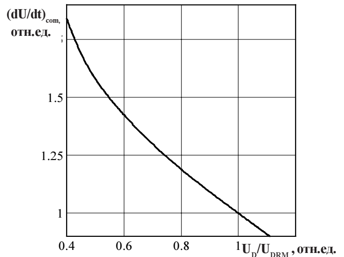
Рисунок 13 - Зависимость критической скорости нарастания коммутационного напряжения (dU_D/dt)_{com} (н.е.д.) от величины приложенного напряжения U_D/U_{DRM} (н.е.д.) при I_T = I_{TRMS} , T_j = 125^\circ\text{C} , t_i = 10\text{ мс} .
