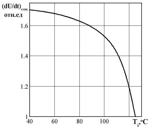
Рисунок 12 - Зависимость критической скорости нарастания коммутационного напряжения (dU_D/dt)_{com} (н.е.д.) от температуры структуры T_j °C при I_T = I_{TRMS} , t_i = 10\text{ мс} .
