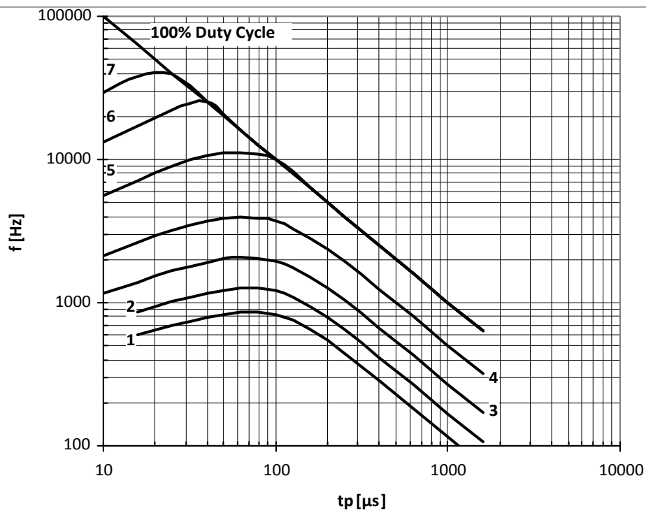
Рис. 12 — Зависимость частоты синусоидальных импульсов тока от длительности импульсов тока
