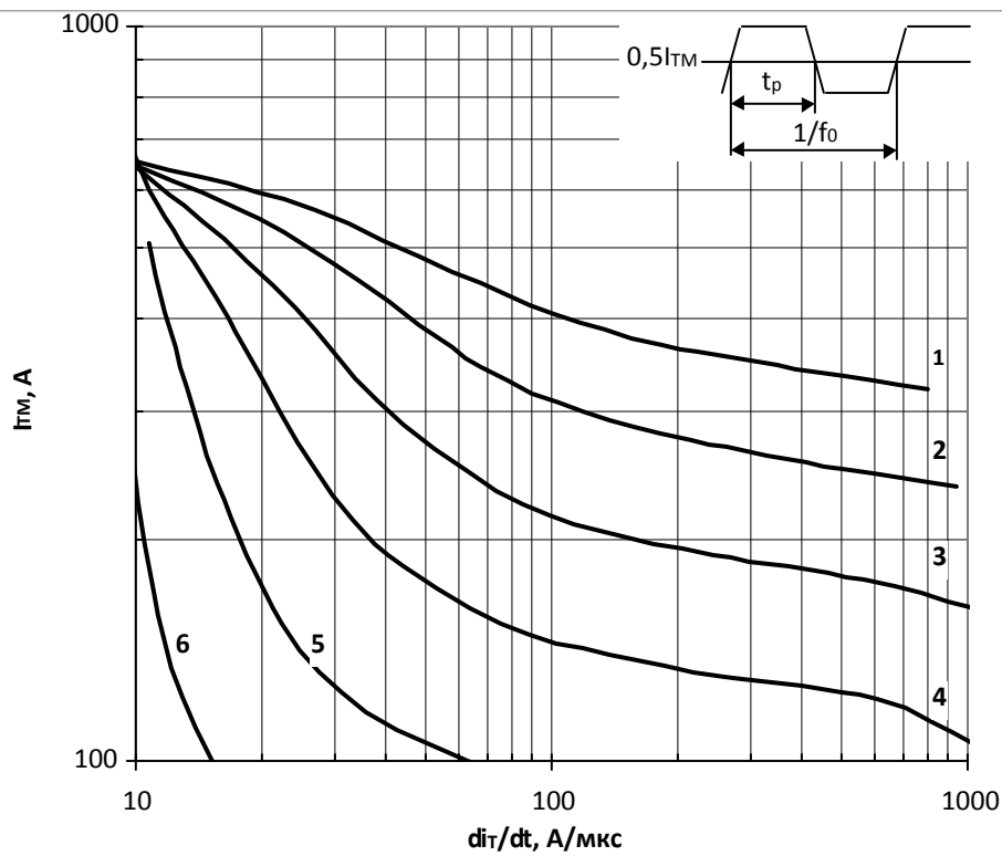
Рис. 15 – Зависимость импульсного тока в открытом состоянии I_{TM} трапециевидной формы тока от скорости нарастания тока di_T/dt для длительности импульсов t_p=1/4f_0 и температуры корпуса T_c=105^\circ\text{C} на высоких частотах.
