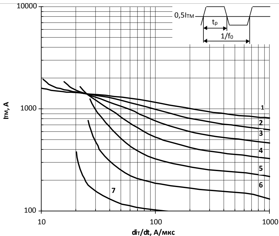
Рис. 13 – Зависимость импульсного тока в открытом состоянии I_{TM} трапециевидной формы тока от скорости нарастания тока di_T/dt для длительности импульсов t_p=1/4f_0 и температуры корпуса T_c=65^\circ\text{C} на высоких частотах.
