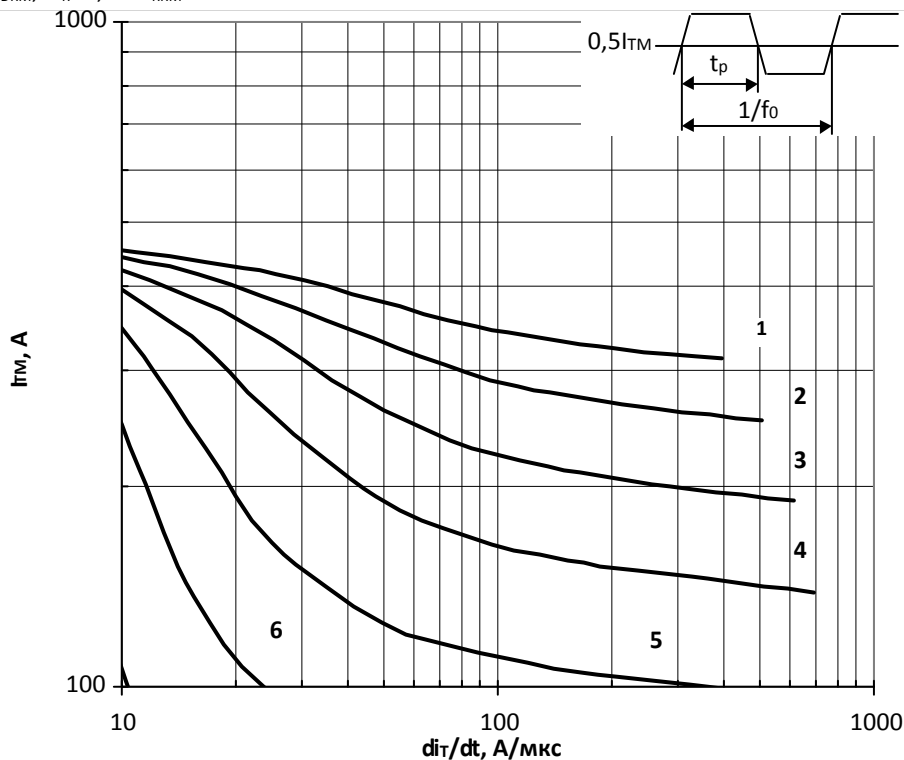
Рис.18 – Зависимость импульсного тока в открытом состоянии I_{TM} трапецевидной формы тока от скорости нарастания тока di_T/dt для длительности импульсов t_p=1/2f_0 , температура охлаждения T_a=40^\circ\text{C} , охлаждающий воздушный поток 6 м/с, радиатор О143 на высоких частотах.
