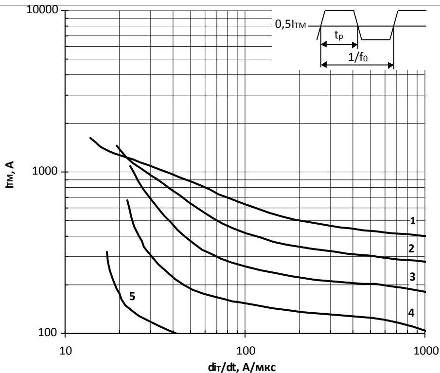
Рис. 17 – Зависимость импульсного тока в открытом состоянии I_{TM} трапецевидной формы тока от скорости нарастания тока di_T/dt для длительности импульсов t_p=1/10f_0 и температуры корпуса T_c=105^\circ\text{C} на высоких частотах.
