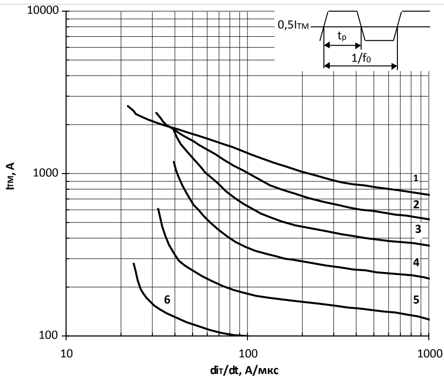
Рис. 16 – Зависимость импульсного тока в открытом состоянии I_{TM} трапециевидной формы тока от скорости нарастания тока di_T/dt для длительности импульсов t_p=1/10f_0 и температуры корпуса T_c=85^\circ\text{C} на высоких частотах.
