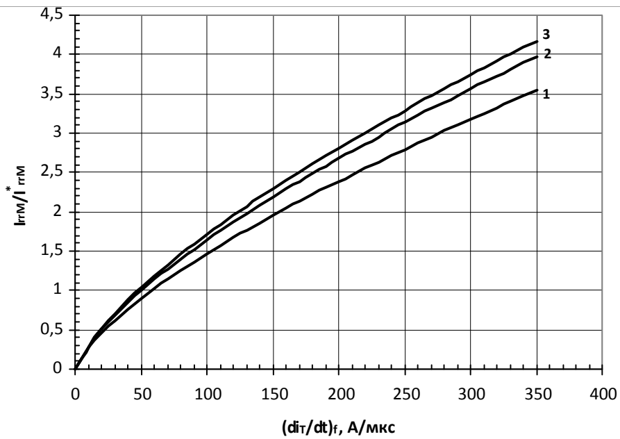
Рис. 33 – Максимальная зависимость тока обратного восстановления I_{rrM} от скорости спада
