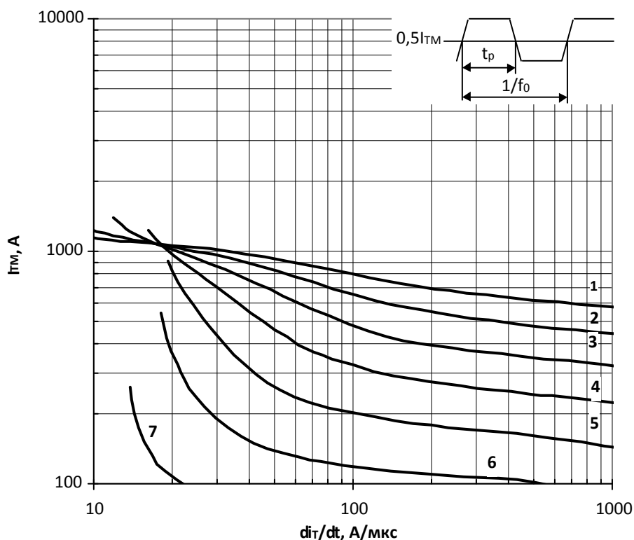
Рис. 14 – Зависимость импульсного тока в открытом состоянии I_{TM} трапециевидной формы тока от скорости нарастания тока di_T/dt для длительности импульсов t_p=1/4f_0 и температуры корпуса T_c=85^\circ\text{C} на высоких частотах.
