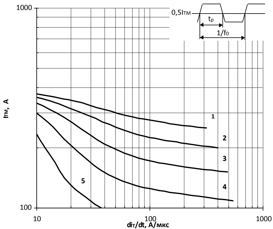
Рис. 12 – Зависимость импульсного тока в открытом состоянии I_{TM} трапециевидной формы тока от скорости нарастания тока di_T/dt для длительности импульсов t_p=1/2f_0 и температуры корпуса T_c=105^\circ\text{C} на высоких частотах.
