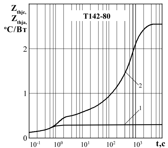
Рисунок 11 - Зависимость теплового сопротивления переход - корпус Z_{thjc} (1) и переход- среда Z_{thja} (2) от времени t при естественном охлаждении T_a = 40\text{ }^\circ\text{C} на типовом охладителе.
