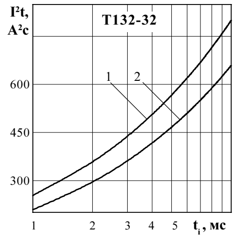
Рисунок 9 - Зависимость защитного показателя I^2t от длительности импульса тока t_i при исходной температуре структуры T_j = 25\text{ °C} (1) и максимальной температуре T_{jm} (2)
