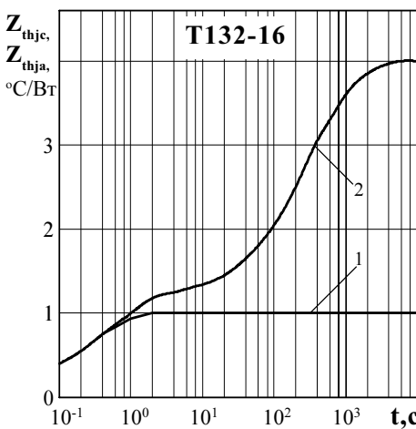
Рисунок 11 - Зависимость теплового сопротивления переход - корпус Z_{thjc} (1) и переход- среда Z_{thja} (2) от времени t при естественном охлаждении T_a = 40\text{ °C} на типовом охладителе.
