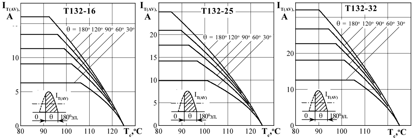
Рисунок 2 - Зависимость допустимого среднего тока в открытом состоянии I_{T(AV)} от температуры корпуса T_c для токов синусоидальной формы частоты f = 50 Гц
