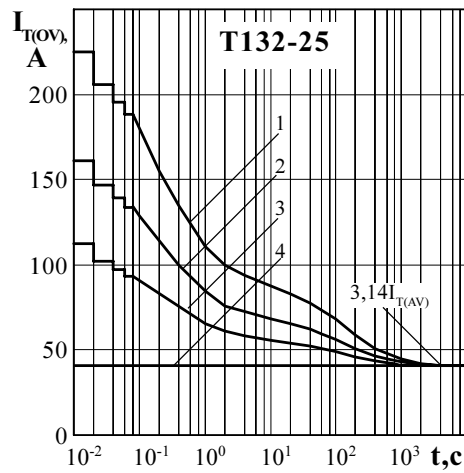
Рисунок 10 - Зависимость допустимой амплитуды тока перегрузки в открытом состоянии I_{T(OV)} синусоидальной формы частотой f = 50\text{ Гц} от длительности перегрузки t при температуре окружающей среды T_a = 40\text{ °C} и при отношении тока, предшествующего перегрузке, I_1 к допустимому среднему току с типовым охладителем I_{T(AV)} равному k = I_T / I_{T(AV)} ; k = 0 (1); 0,5 (2); 0,75 (3); 1,0 (4).
