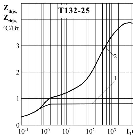
Рисунок 11 - Зависимость теплового сопротивления переход - корпус Z_{thjc} (1) и переход- среда Z_{thja} (2) от времени t при естественном охлаждении T_a = 40\text{ °C} на типовом охладителе.
