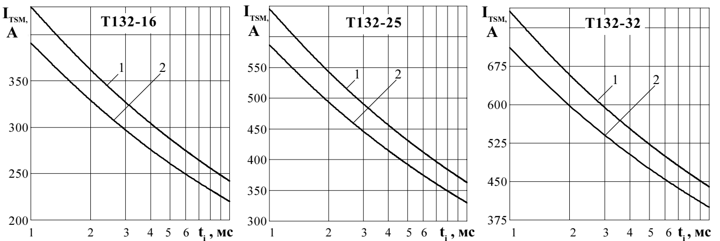
Рисунок 8 - Зависимость допустимой амплитуды ударного тока в открытом состоянии I_{TSM} от длительности импульса тока t_1 при исходной температуре структуры T_j = 25 °C (1) и максимальной температуре T_{jm} (2)
