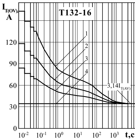
Рисунок 10 - Зависимость допустимой амплитуды тока перегрузки в открытом состоянии I_{T(OV)} синусоидальной формы частотой f = 50\text{ Гц} от длительности перегрузки t при температуре окружающей среды T_a = 40\text{ °C} и при отношении тока, предшествующего перегрузке, I_1 к допустимому среднему току с типовым охладителем I_{T(AV)} равному k = I_T / I_{T(AV)} ; k = 0 (1); 0,5 (2); 0,75 (3); 1,0 (4).
