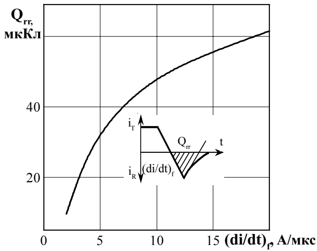
Рисунок 17 - Зависимость заряда восстановления ления Q_{rr} от скорости спада тока (di/dt)_f в открытом состоянии при температуре перехода T_{jm} = 125^\circ\text{C} , U_{RM} = 100\text{ В} ; I_T = I_{T(AV)} .
