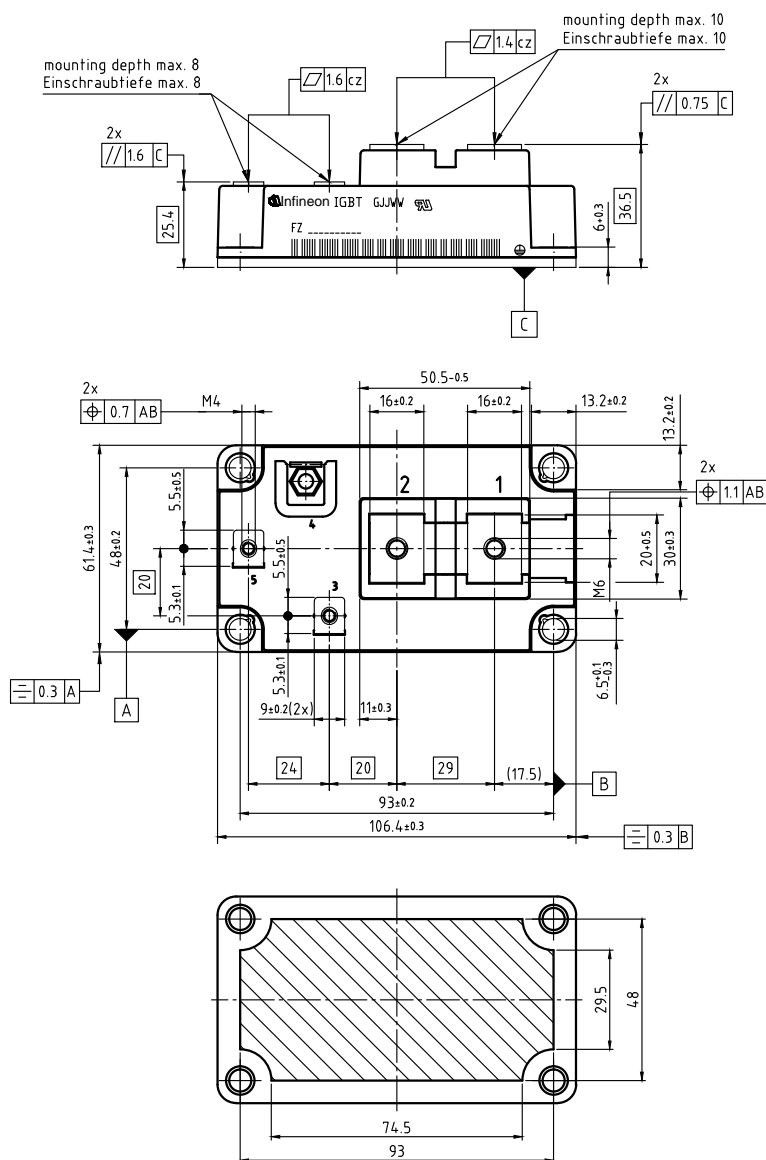
Sperrfläche für Thermisches Interface Material restricted area for Thermal Interface Material
